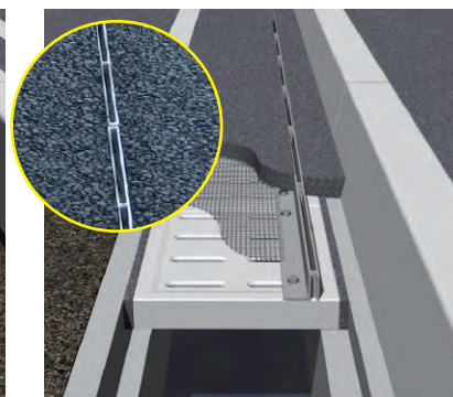
スリット幅9mmタイプ
