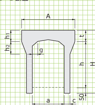
■B-B'断面
