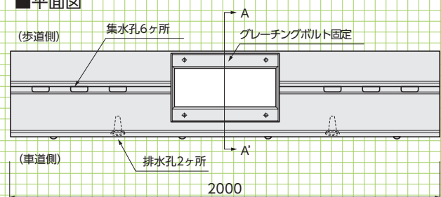
■平面図
