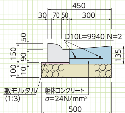
■乗入部断面図
