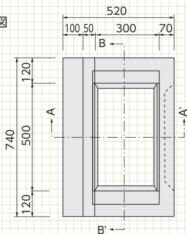
■A-A'断面図
