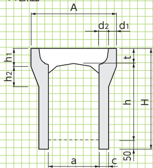
■A-A'断面
