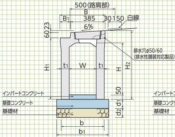
■断面図 (W=300,400)
