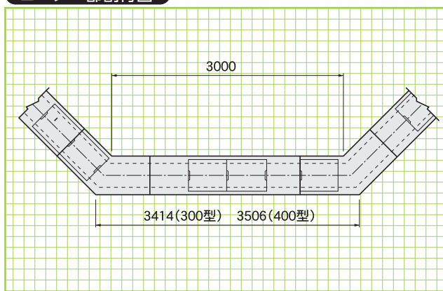
コーナー部割付図
