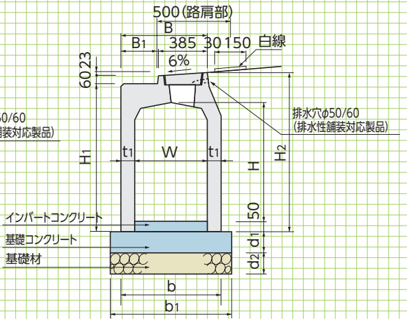
■断面図 (W=500,600)
