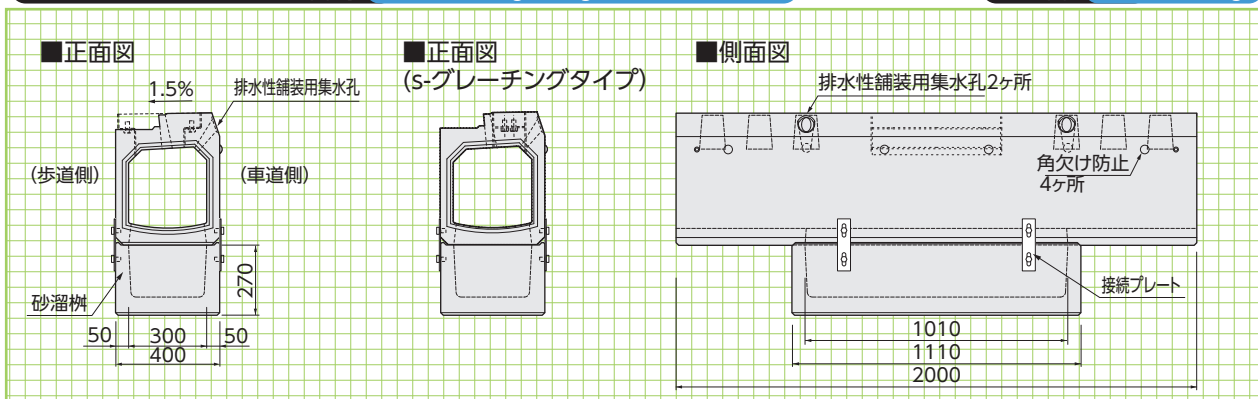
縦断400グレーチング砂溜柵用 参考重量:600kg/614kg(s-グレーチングタイプ)
