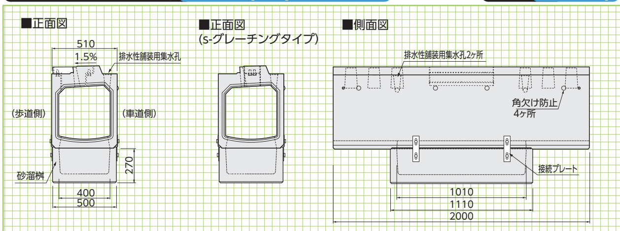
縦断400グレーチング砂溜柵用 参考重量:600kg/614kg(s-グレーチングタイプ)
