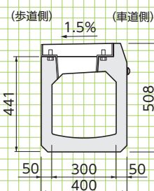
■A-A'断面図
