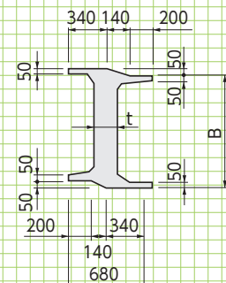
■A-A'断面図
