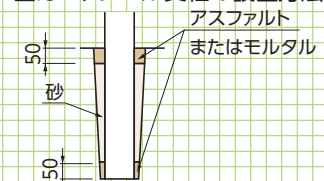
■B-B'断面図
