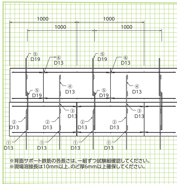
■背面側セット状況
