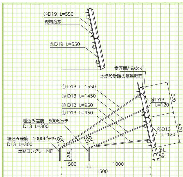
■背面サポート参考断面図
