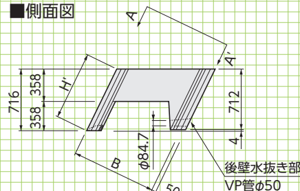
■側面図
