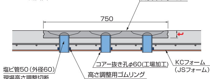
■A-A'断面図
